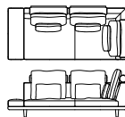
S-581L 2人掛けコーナーソファ + アーム W2365×D1055×H830×SH380
