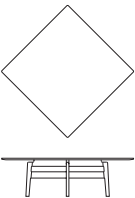
T-875 ダイニングテーブル W1800×D1800×H730
