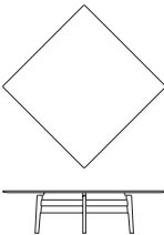
T-876 ダイニングテーブル W2000×D2000×H730
