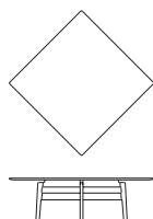
T-875 dining table W1800×D1800×H730
